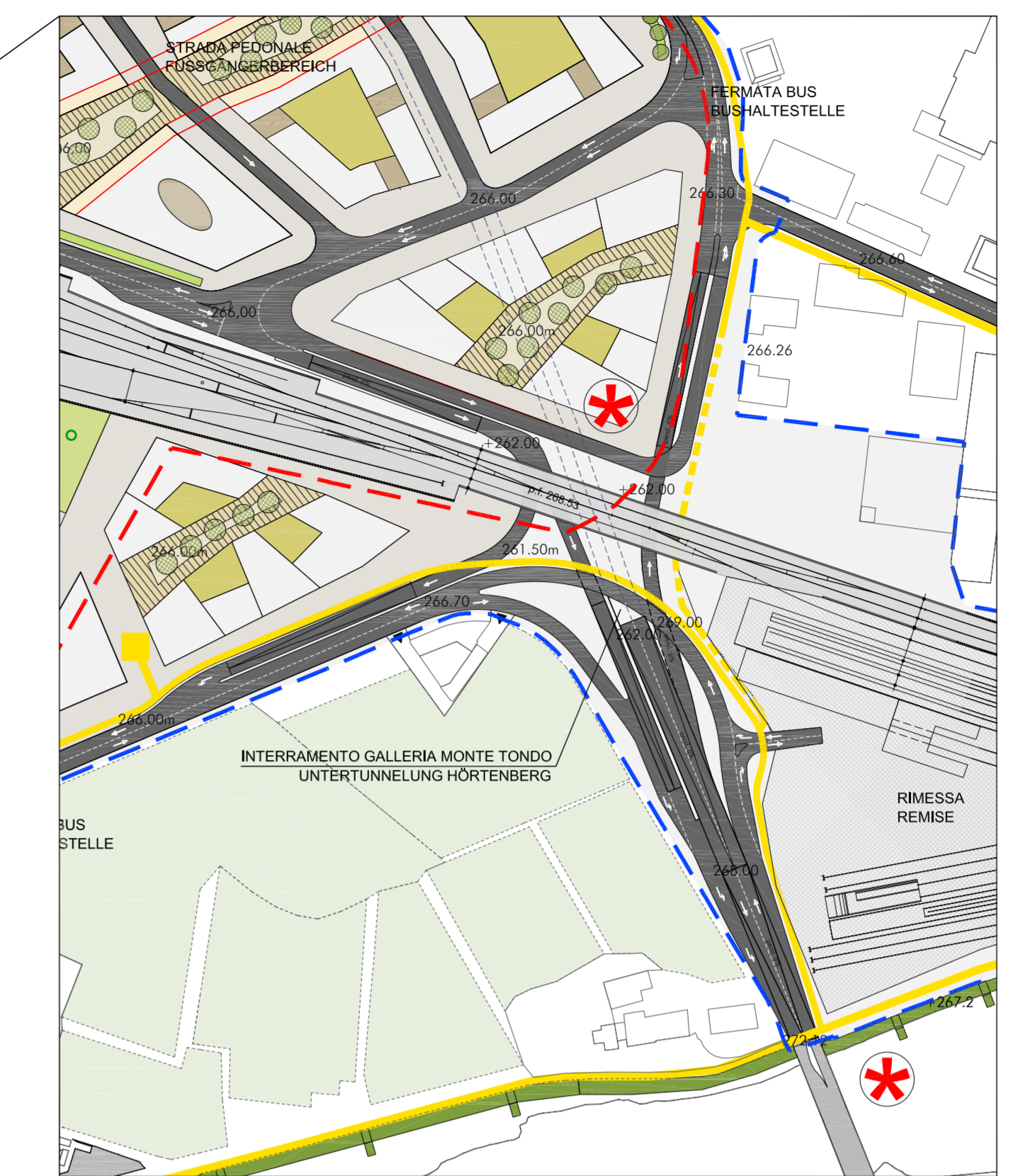
STUDIO B - SVINCOLO CON STUDIO INSERIMENTO TUNNEL DEL MONTE TONDO STUDIE B - ANSCHLUSS MIT EINFÜGUNG DES HÖRTENBERGTUNNELS
