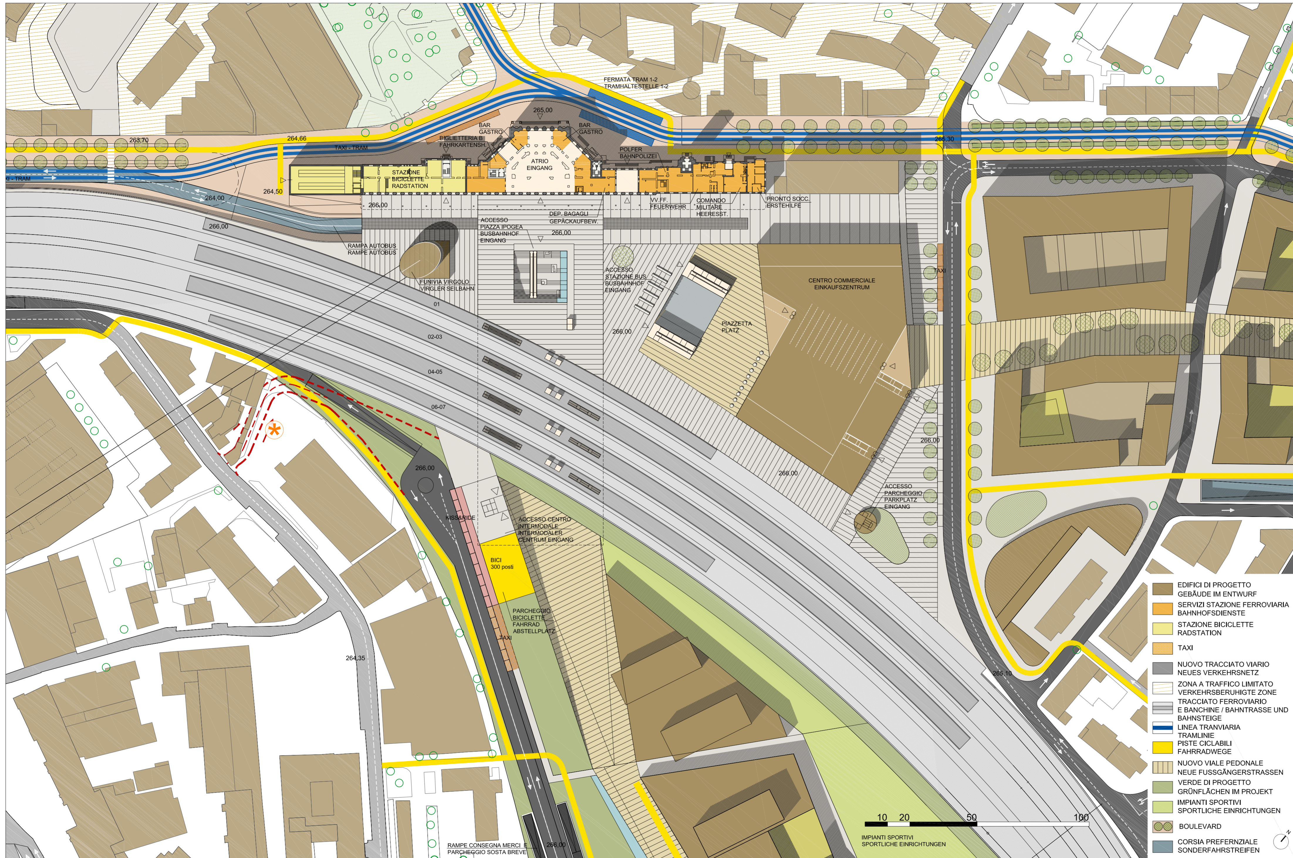
Pianta livello 0 / Grundriss Niveau 0 scala / Masstab 1:1000
